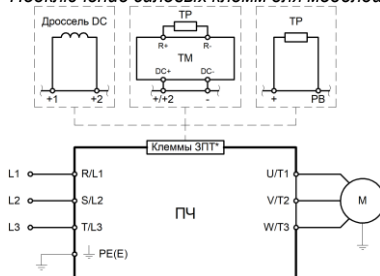
Рис. 3.2.4 — Подключение силовых клемм для моделей LCI-GY/PY-4(B)
