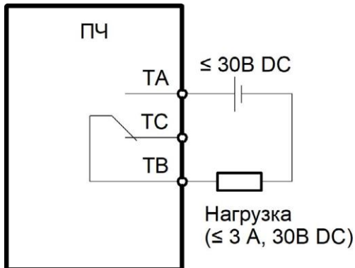
Рис. 3.12 – Схема подключения нагрузки постоянного тока к релейному выходу
