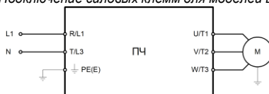
Рис. 3.2.3 — Подключение силовых клемм для моделей LCI-GY/PY-3
