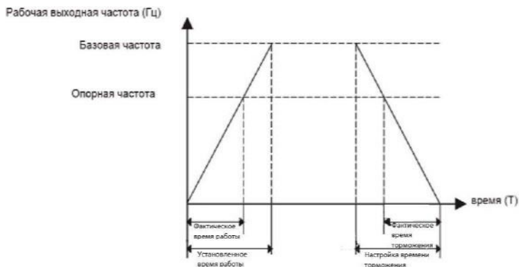
Рис. 6.1 - Время разгона/торможения
