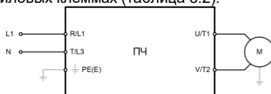
Рис. 3.2.1 — Подключение силовых клемм для моделей LCI-GY/PY-1
