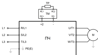
Рис. 3.2.5 — Подключение силовых клемм для моделей LCI-GY/PY-6
