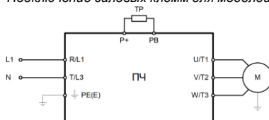
Рис. 3.2.2 — Подключение силовых клемм для моделей LCI-GY/PY-2(B)
