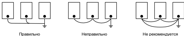
Рис. 3.5 — Схематичное изображение образования петли с заземляющим проводом
